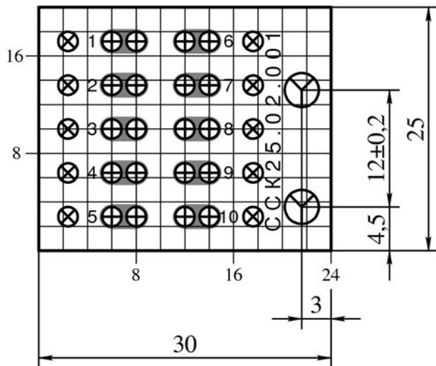
Сторона установки элементов
